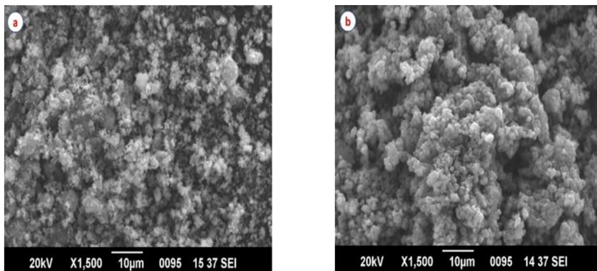
Fig. 5. SEM images for (a) TiO_2 nanoparticles and (b) TiO_2 -PANI nanocomposite
